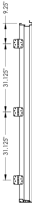
HINGE JAMB
